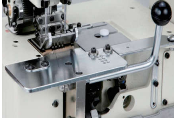
■ TB ターンダウンホルダーブラケット (*1508SPF,1509SPFは標準装備) TURN DOWN FOLDER BRACKET (*This is standard equipment for 1508SPF,1509SPF.) EQUIPAMENTO ESTANDAR (PARA 1508SPF, 1509SPF) 拉开式面板 (1508SPF,1509SPF 标准装备)
