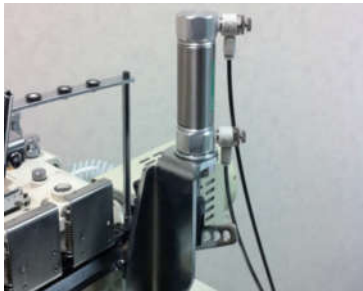
■ FL エアー式押え上装置 AIR TYPE FOOT LIFTER FL: LEVANTA PIE NEUMATICO 气压式抬压脚装置
